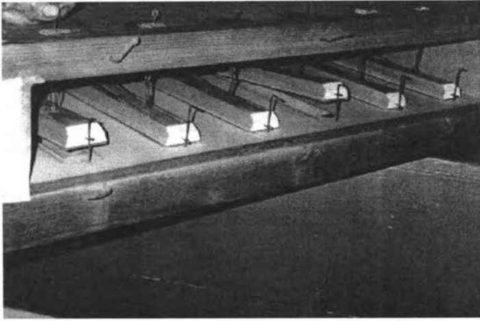
Mechanikus orgona, szelepek
