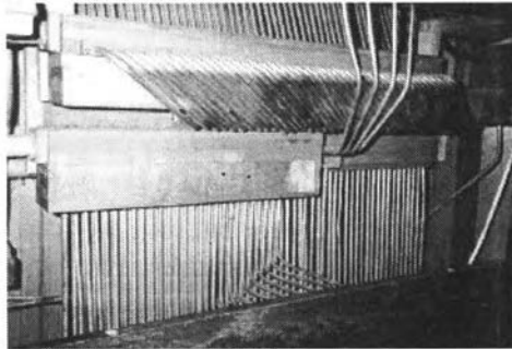
Pneumatikus orgona belseje, ólomcsövek
