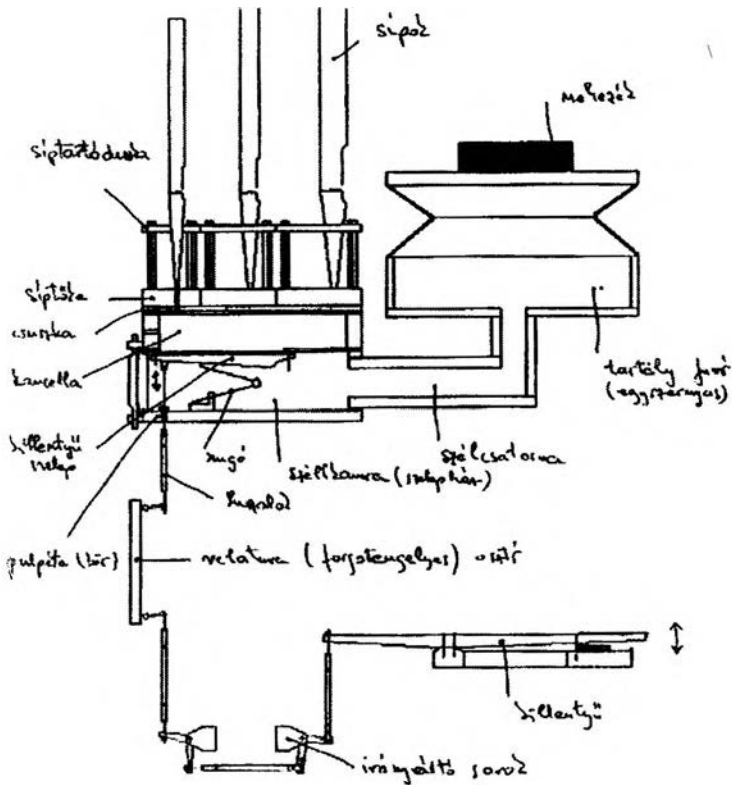
Mechanikus orgona szerkezete, Molnár József rajza
