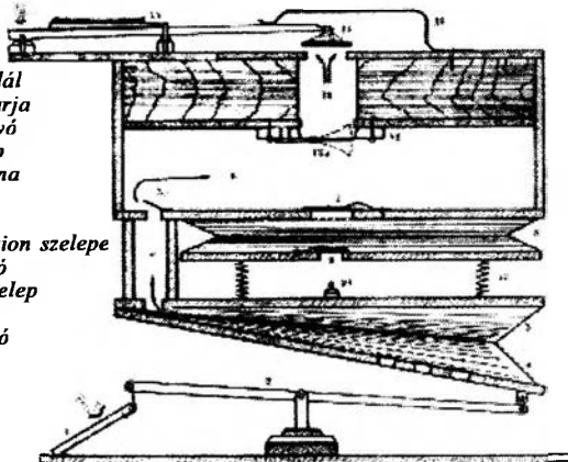
A fúvólégrendszerű harmónium (2)
