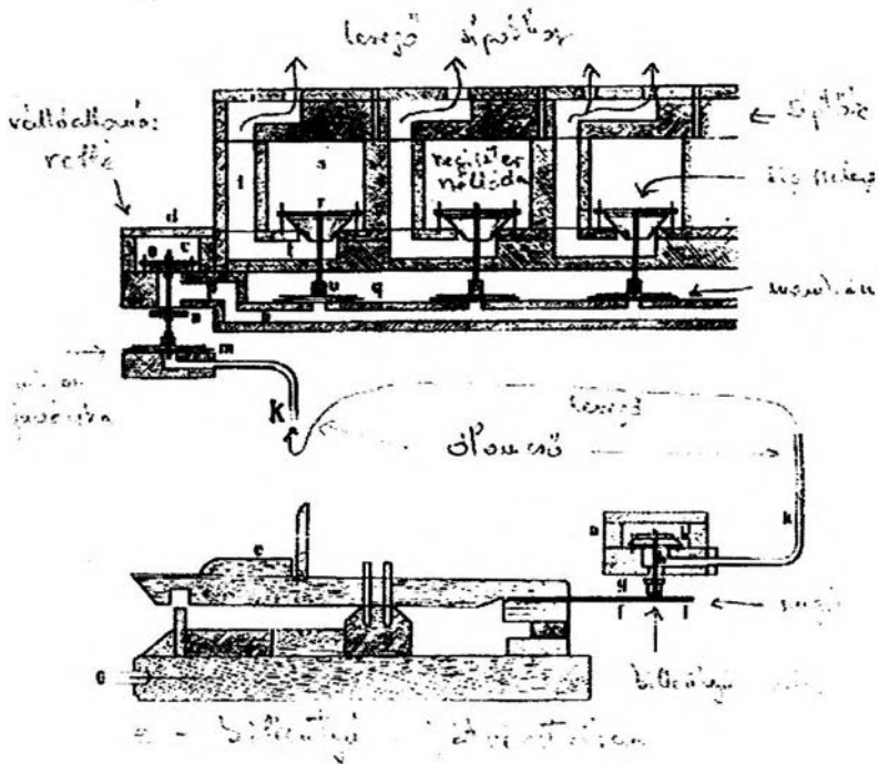
Pneumatikus orgona szerkezete, Molnár József rajza
