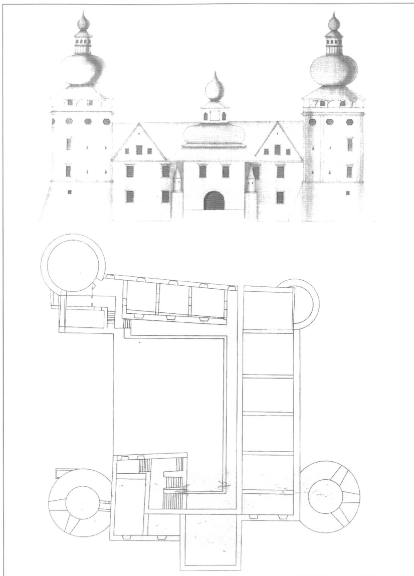
A 18. századi kastély, a főhomlokzat felmérési és az első emelet alaprajza. [1783MOL Tervtár.I. 20.99/4]
